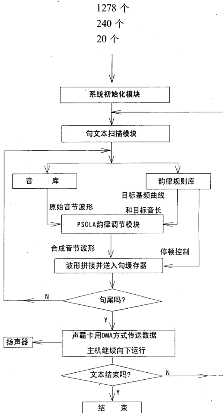
图1 基于PSOLA技术的波形拼接 汉语文语转换系统的流程图
